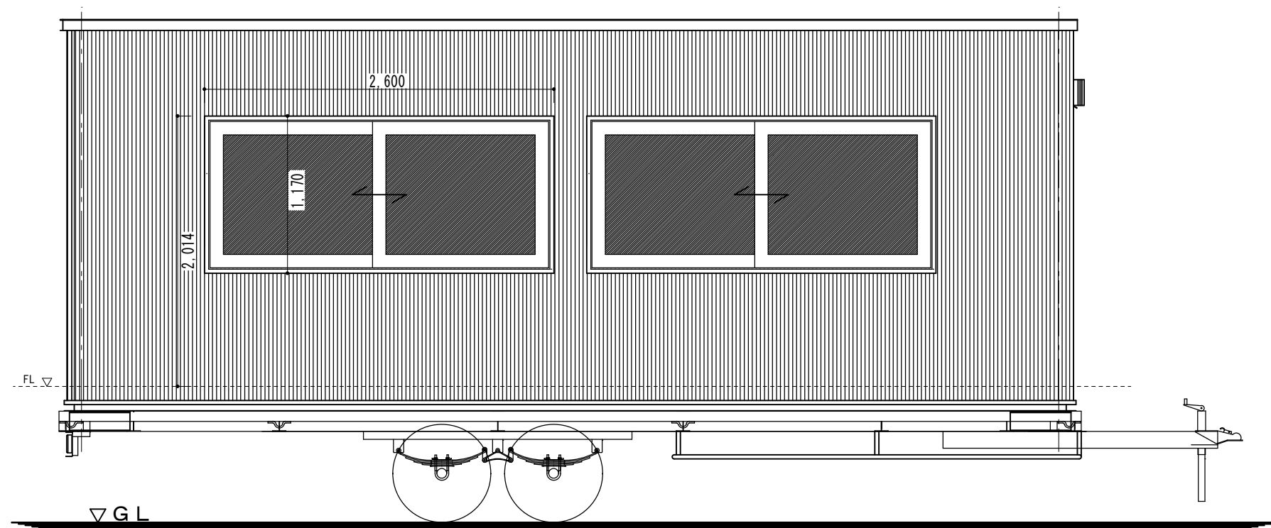
南立面图
