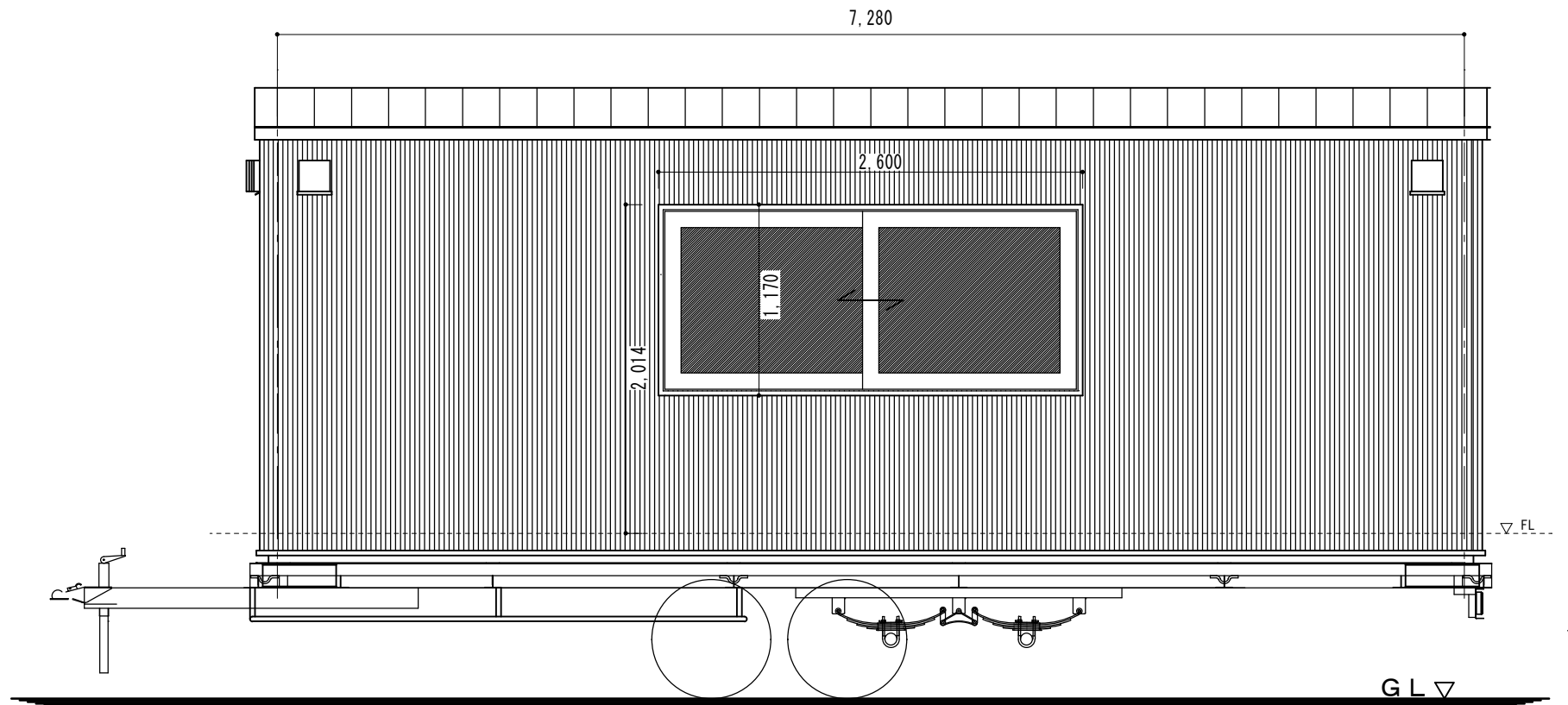
北立面图
