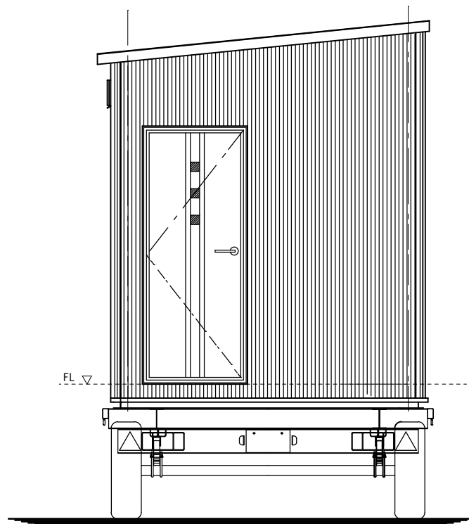
西立面图
