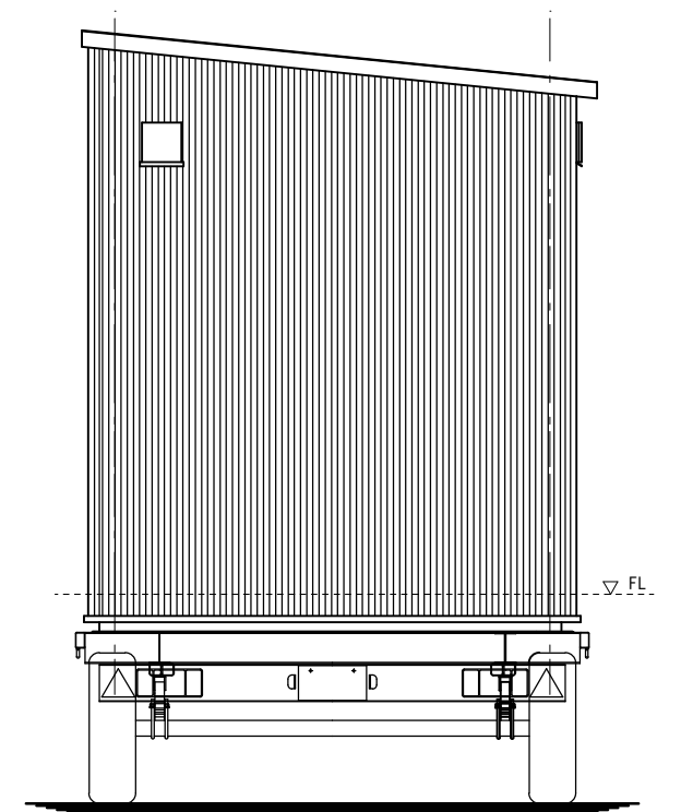
東立面图
